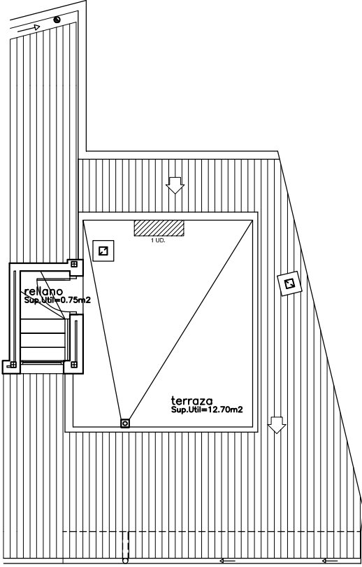
CUBIERTA VIVIENDA 7
