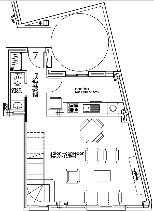
PLANTA PRIMERA. VIVIENDA 7
